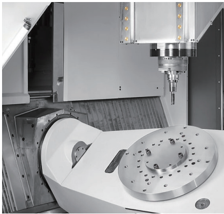
FZ 25 S five axis 加工区域
