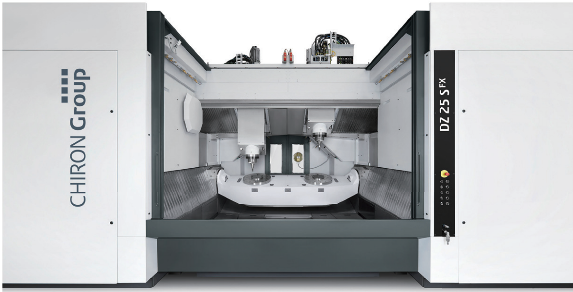
DZ 25 S five axis 双主轴五轴加工中心 主轴间距为 800mm, 可在 X 轴与 Z 轴方向独立运动。
